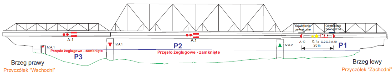
Rysunek 2 Ruch żeglugowy zachodnim przęsłem
