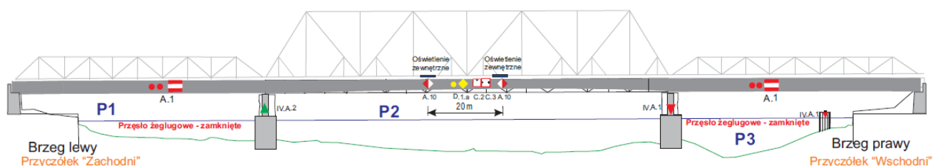
PRZEPRAWA MOSTOWA w km 734,6 rz. Regalicy (widok na most drogowy od strony wody górnej)
