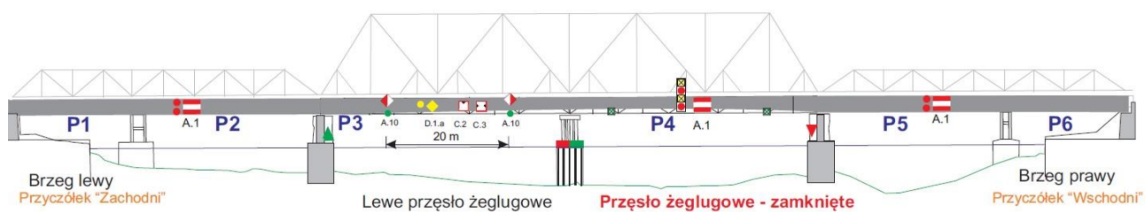
PRZEPRAWA MOSTOWA w km 734,6 rz. Regalicy (widok na most kolejowy od strony wody dolnej)
